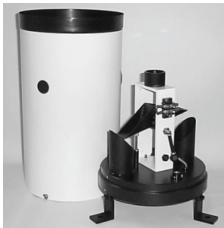
Pluviômetro
